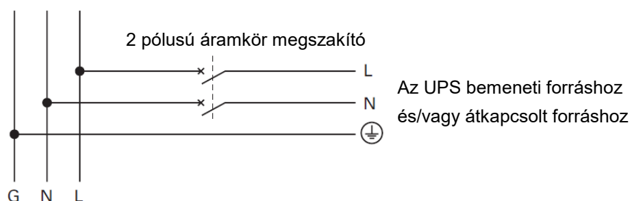
8. ábra. Bemeneti védelem
