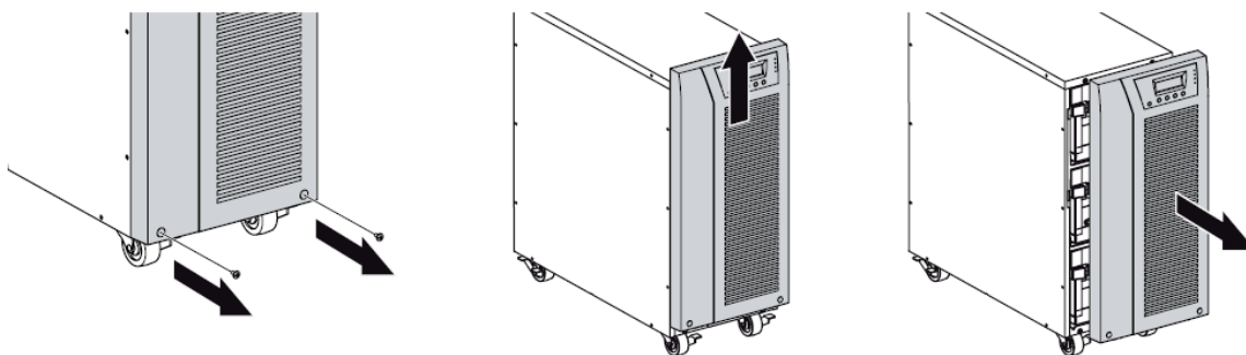
27. ábra. Az UPS előlap eltávolítása
